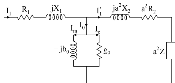
● 等效至一次側電路 ●
