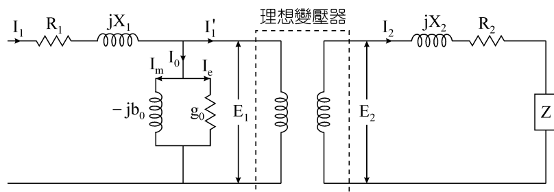
● 變壓器等效電路 ●
